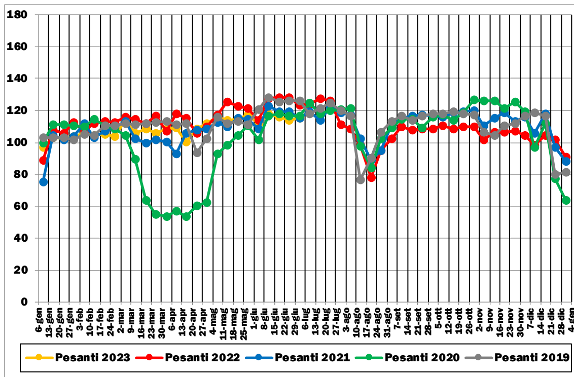
FIGURA 2.28: TRAFFICI STRADALI GIORNALIERI MEDI PESANTI (GENNAIO 2019-GIUGNO 2023)
